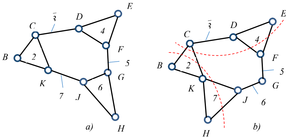
Şəkl. 5. a) Altıncı sinfə mənsub üçtərtibli Assur qrupu ( s=6, n=6, p=9, t=3, c=0 ); b) Sərbəstlik dərəcəsi sıfıra bərabər olan kinematik silsilə
