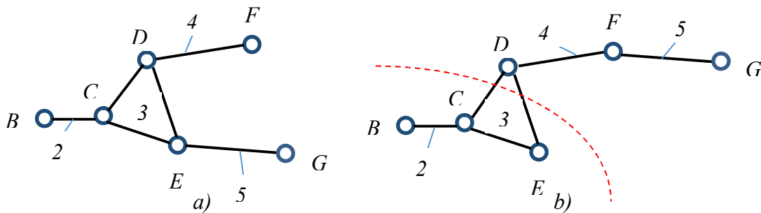
Şək. 2. a) Üçüncü sinfə mənsub üçtərtibli (üçcilovlu) Assur qrupu ( s=3, k=4, p_s=6, t=3, c=3 ); b) Sərbəstlik dərəcəsi sıfıra bərabər olan kinematik silsilə
