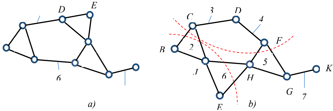
Şəkl. 4. a) Beşinci sinfə mənsub üçtərtibli (bircilovlu) Assur qrupu ( s=5, n=6, p=9, t=3, c=1 ); b) Sərbəstlik dərəcəsi sıfıra bərabər olan kinematik silsilə
