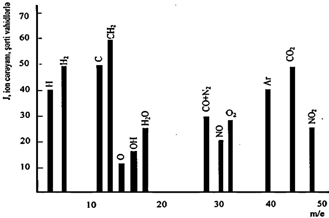
Şək. 2. Polietilen materialına oksigen mühitdə səyriyyən qazboşalmasının təsirini xarakterizə edən kütlə spektroqramı
