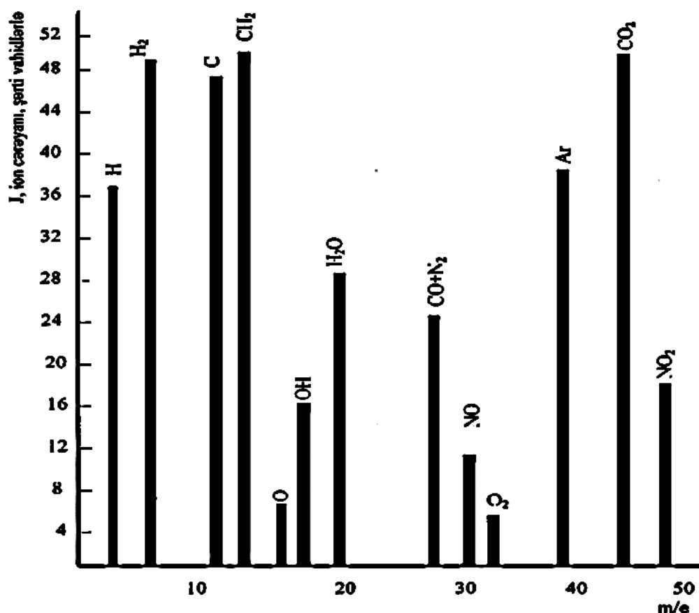
Şəkl. 1. Polietilen materialına səyriyən qazboşalmasının təsirini xarakterizə edən kütlə spektroqramı
