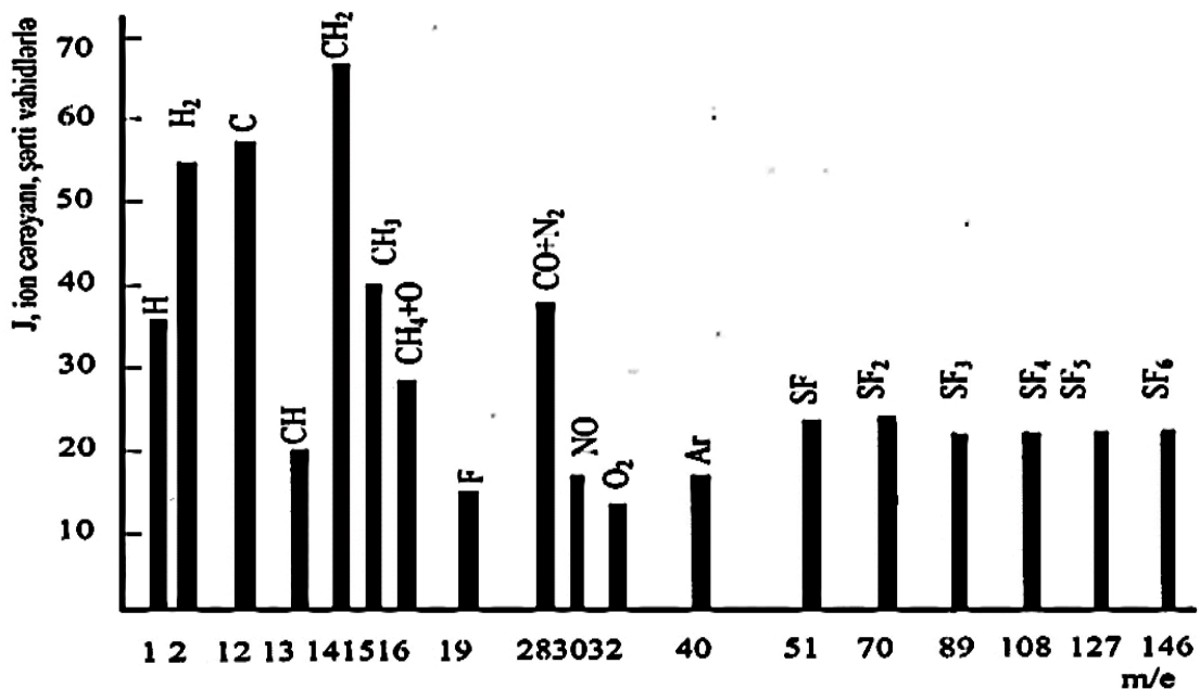
Şək. 3. Polietilen materialına SF_6 qazı mühitinin səyriyyən qazboşalmasının təsirini xarakterizə edən kütlə spektroqramı
