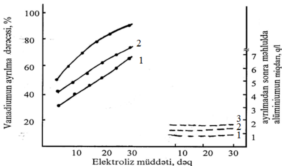
Şəkl. 1. Məhlullardan vanadiumun qallam elektrodunda reduksiyasına temperaturun təsiri
